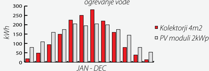
Letni neto donos energije toplotnih in fotonapetostnih SSE za ogrevanje vode
